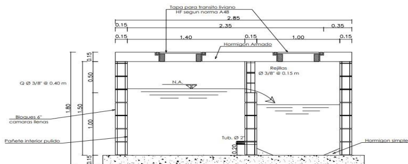
B-B
